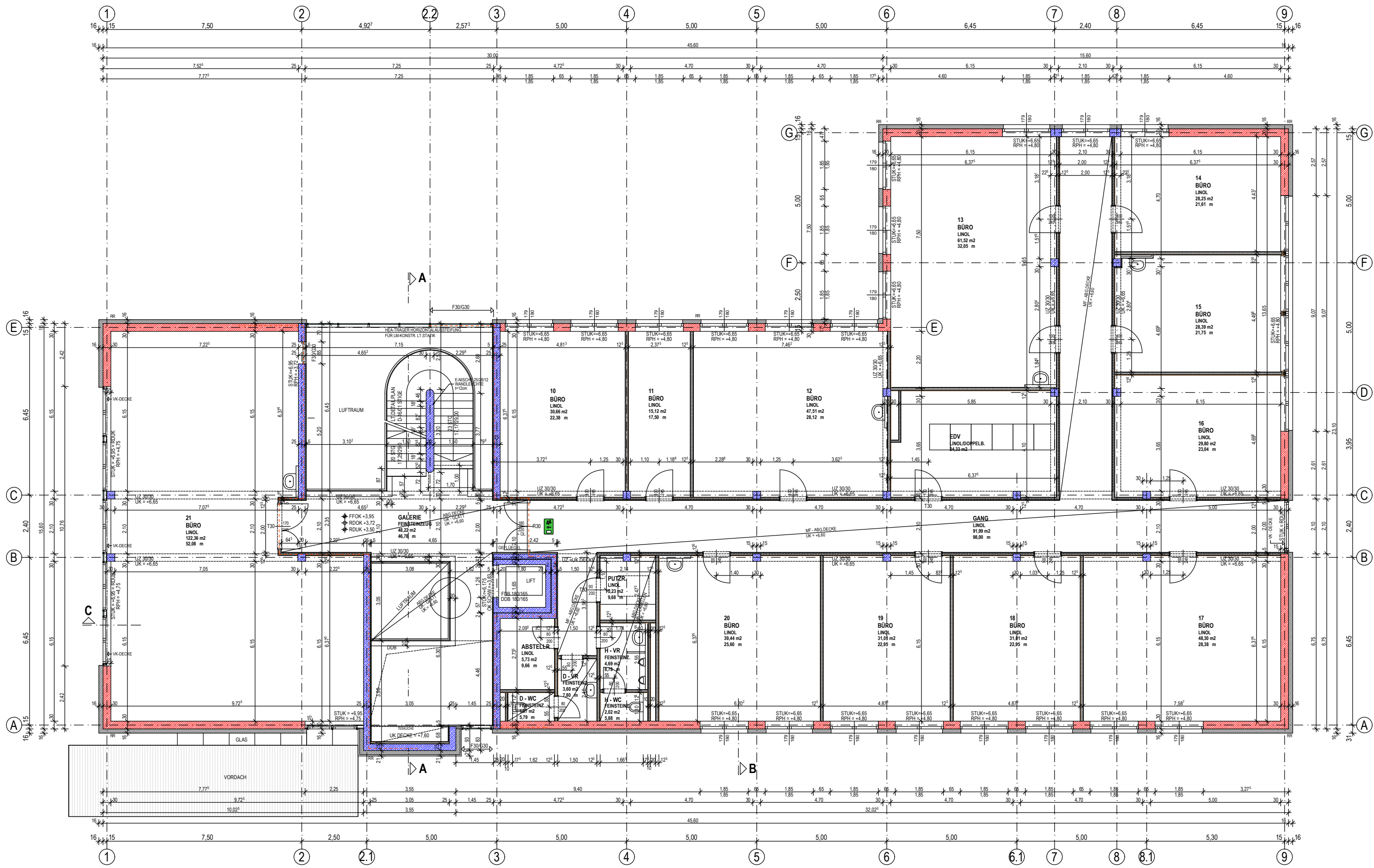
TZ MONDSEELAND - 1.OBERGESCHOSS
